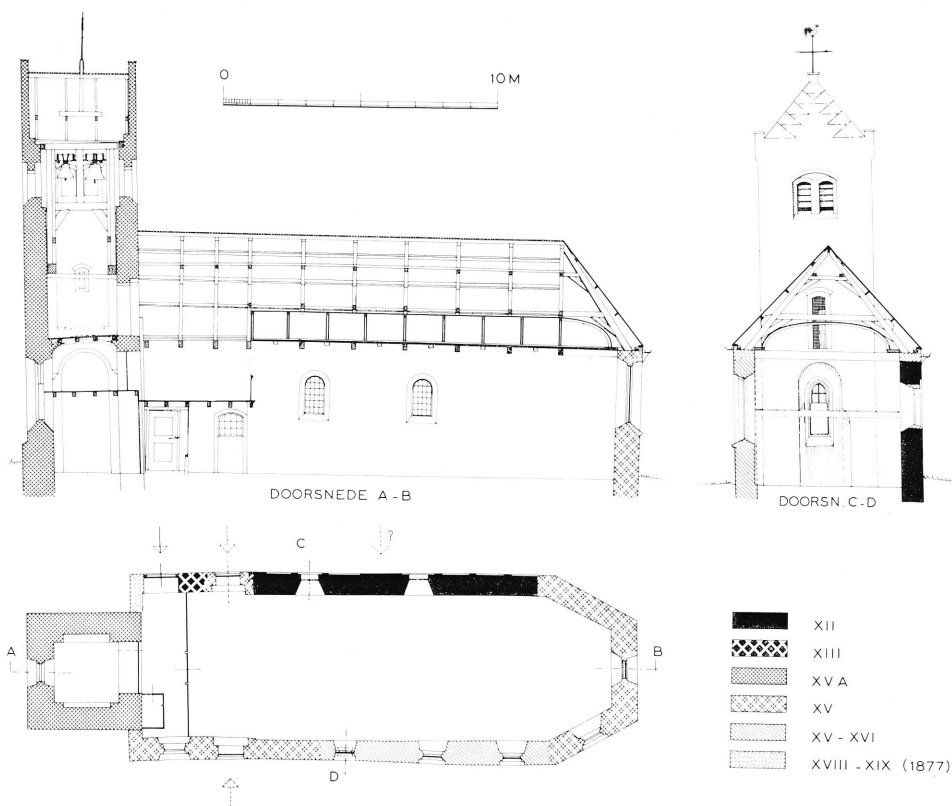
Ned. Herv. kerk Genum. (Tekening W. J. Berghuis, 1972, naar opmetingen van H. v. d. Wal, 1944.)
