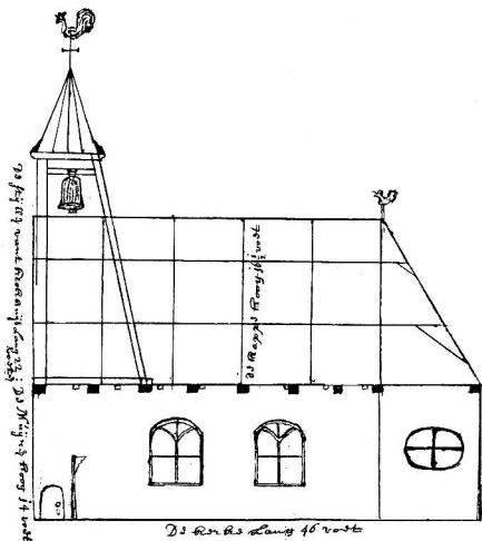
9. Bestektekening van de kerk van Sandfirden uit 1732 (gem. archief Wymbritseradeel). Ook de kerken van Spannum (1742) en Westhem (1708) hebben in het koor een dergelijk raam.
