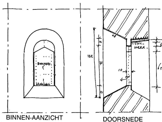
DOORSNEDE
