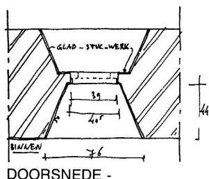
DOORSNEDE -
