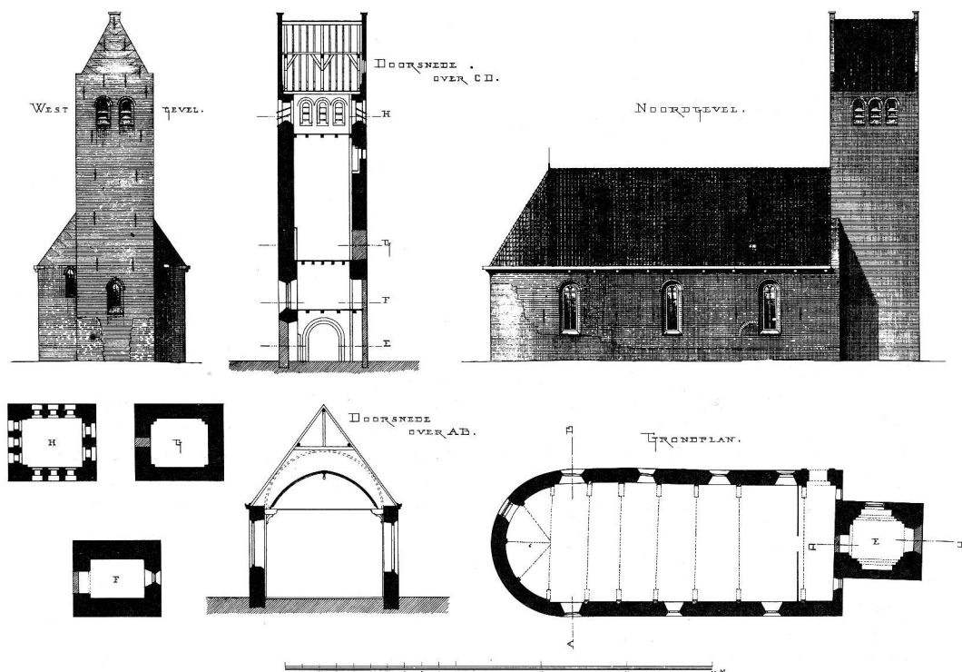
4. Uitgewerkte bouwkundige tekening door A. Mulder, 1883. Coll. R.D.M.Z. te Zeist.
