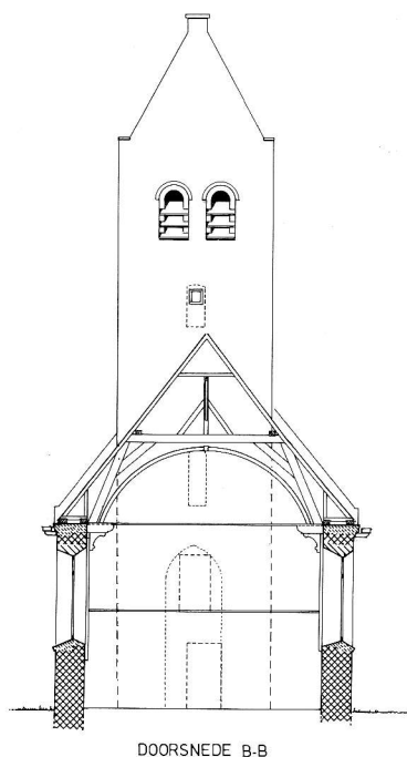
DOORSNEDE B-B
