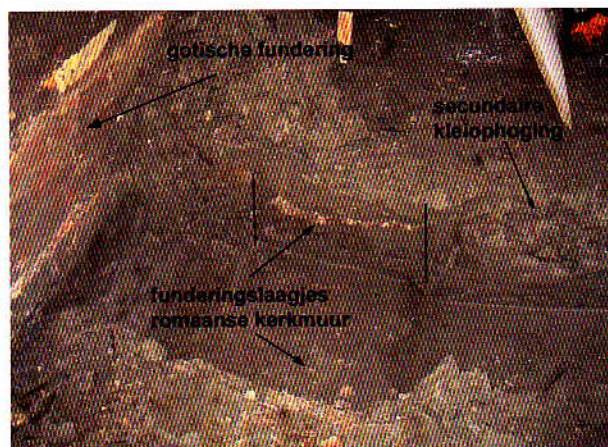
Op circa 50 cm uit de zuidgevel kwam een oude funderingsaanleg tevoorschijn. De laagjes bestaan uit afwisselend klei en baksteenpuin
