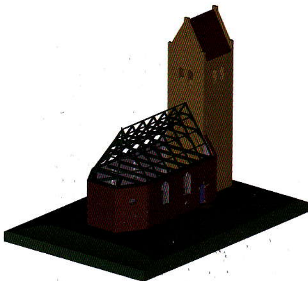
Reconstructie van de situatie in 1708, waarbij het dakbeschot en de pannen zijn weggelaten. Let op de kap en de vensters
